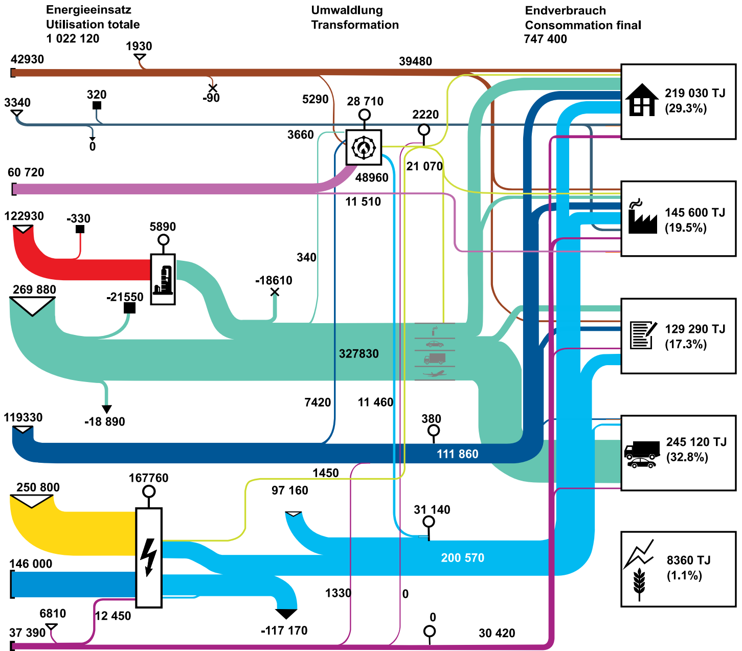
Fig. 5 Detailliertes Energieflussdiagramm des Schweiz 2020 (in TJ) Flux énergétique détaillé de la suisse en 2020 (en TJ)
